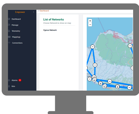
Front-end εφαρμογής
